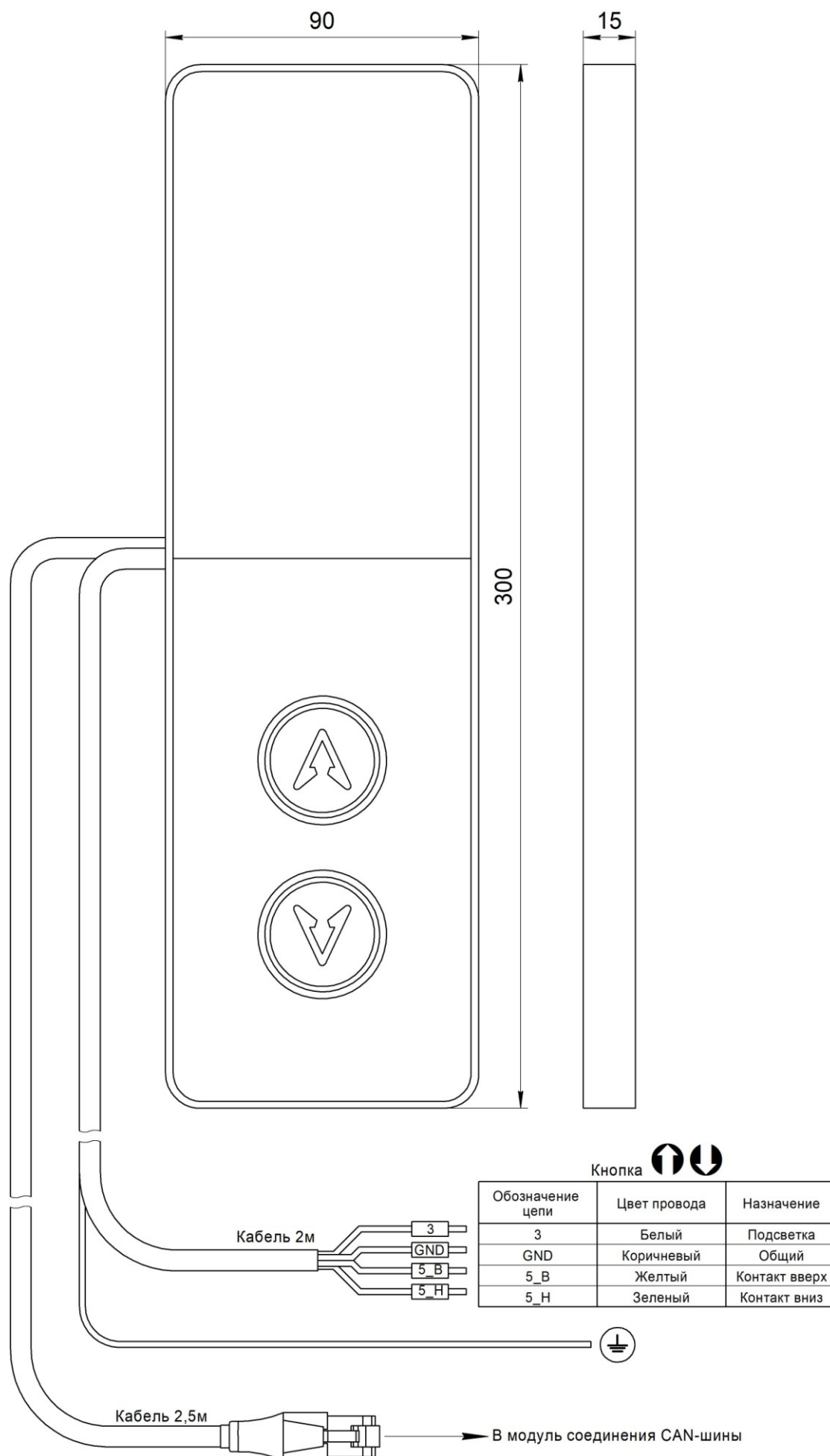
Рис.1 Внешний вид Вызывной пост ОПАЛ (жгут RJ45) НШЕК.468381.057
